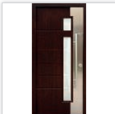
AFB. Drzwi wejściowe zewnętrzne model 437,1 systemu E-82. Wymiary zewnętrzne ościeżnicy [cm]: 98/209. Grubość [mm]: 82. Wyposażenie: zamek listwowy klasy „C” na dwie wkładki, 4 kołki antywłamaniowe. Szklenie: pakiet 3 szybowy z szybą niskoemisyjną P1. Materiał: klejone warstwowo drewno mahoń-meranti. Ocieplenie [mm]: 58. Współczynnik przenikania ciepła U_d [W/(m 2 K)]: 0,7. Gwarancja: 4 lata. Cena netto [zł]: 4366.
