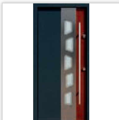
AFB. Drzwi wejściowe zewnętrzne model 451,1 systemu E-82. Wymiary zewnętrzne ościeżnicy [cm]: 98/209. Grubość [mm]: 82. Wyposażenie: zamek listwowy klasy „C” na dwie wkładki, 4 kołki antywłamaniowe. Szklenie: pakiet 3 szybowy z szybą niskoemisyjną P1. Materiał: klejone warstwowo drewno mahoń-meranti. Ocieplenie [mm]: 58. Współczynnik przenikania ciepła U_d [W/(m 2 K)]: 0,7. Gwarancja: 4 lata. Cena netto [zł]: 4366.
