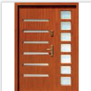
AFB. Drzwi zewnętrzne dwuskrzydłowe model 911,1 systemu E-82. Wymiary zewnętrzne ościeżnicy [cm]: 148/209. Grubość [mm]: 82. Wyposażenie: zamek listwowy klasy „C” na dwie wkładki, 4 kołki antywłamaniowe. Szklenie: pakiet 3 szybowy z szybą niskoemisyjną P1. Materiał: klejone warstwowo drewno mahoń-meranti. Ocieplenie [mm]: 58. Współczynnik przenikania ciepła U_d [W/(m 2 K)]: 0,7. Gwarancja: 4 lata. Cena netto [zł]: 6998.
